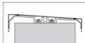
内勾配笠木(見付60mm)
